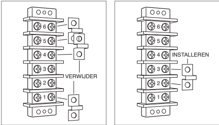
3-fasig
