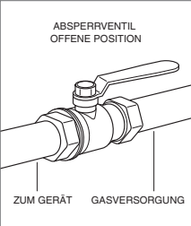
Gasabsperrventil
