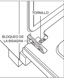
Extracción de la puerta del horno
