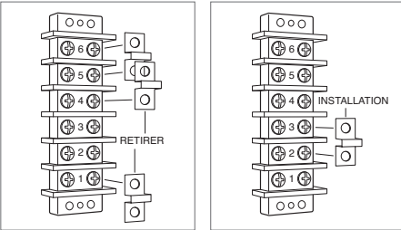
Triphasé
