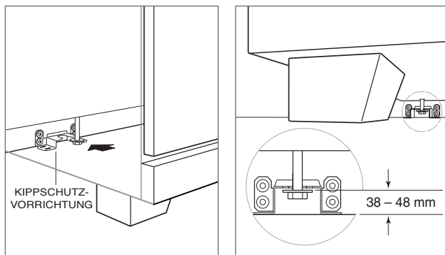
Position der Kippschutzvorrichtung
