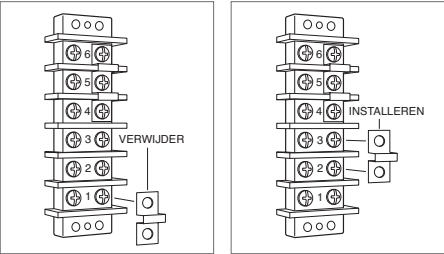
1-fasig
