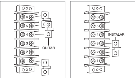
Cableado trifásico
