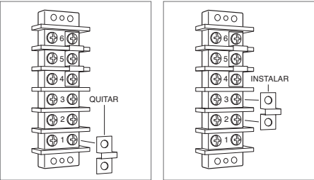
Cableado monofásico
