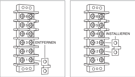
Einphasig Einphasig
