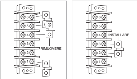
Trifase
