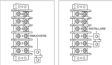
Monofase
