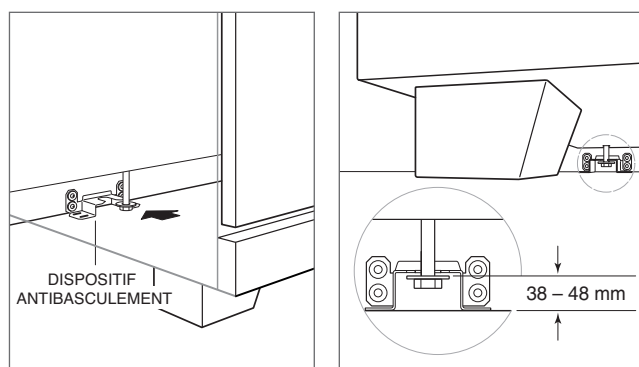
Emplacement du support antibasculement.
