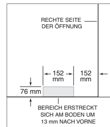
Ort der Wasserversorgung (ICBW-30CI)
