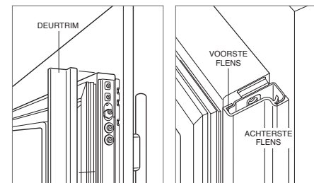
Deurtrim.
