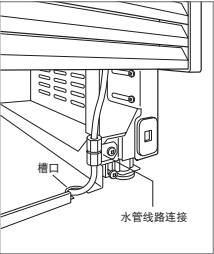
水管线路(ICBIW-30CI)。
