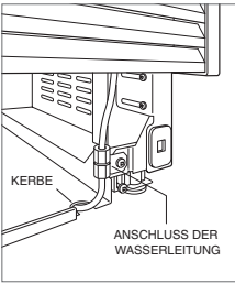
Wasserleitung (ICBW-30CI)
