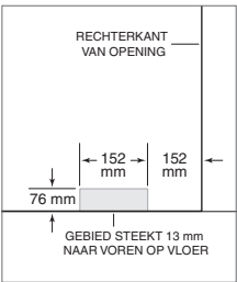
Locatie watertoevoer (ICBIW-30CI).
