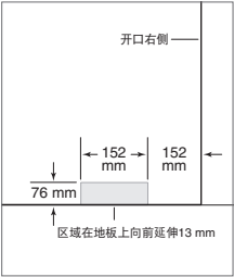
供水位置(ICBIW-30CI)。
