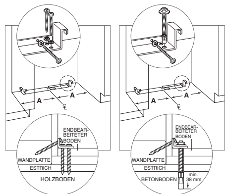
Holzboden
