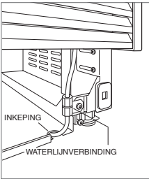
Waterleiding (ICBIW-30CI).
