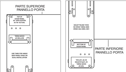
Dima pannello porta, parte superiore. Dima pannello porta, parte inferiore (solo modelli alti).
