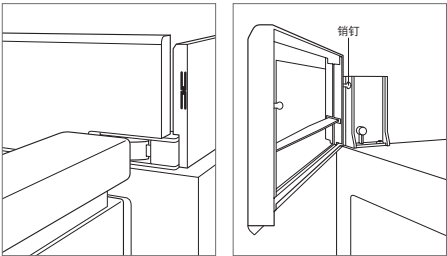
顶饰—铰链侧。顶饰安装—手柄侧。
