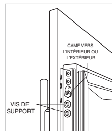
Ajustement vers l'intérieur ou l'extérieur.
