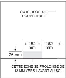
Emplacement de l'arrivée d'eau (dessous).
