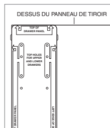
Gabarit pour les panneaux de tiroir - dessus.
