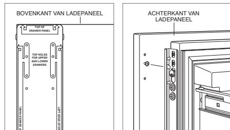
Sjabloon ladepaneel: bovenkant.
