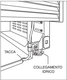
Linee acqua (ICBW-30CI).
