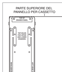
Dima pannello cassetto, parte superiore.
