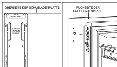
Schubladenplattenvorlage – oben.
