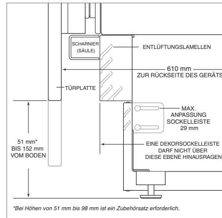
Sockelleiste (Seitenansicht)
