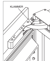
Türanschlag von 90°
