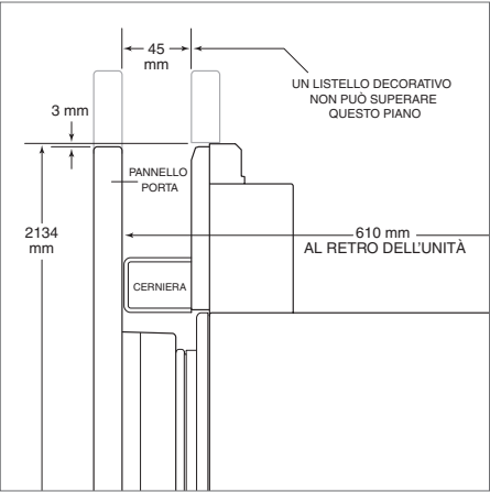
Listello superiore (vista laterale).
