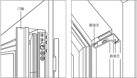
门饰。
