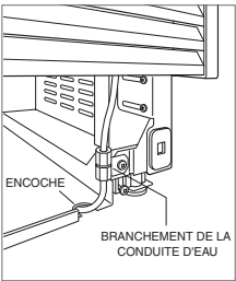
Canalisation d'eau (ICBIW-30CI).
