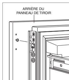
Fixation des panneaux de tiroir.
