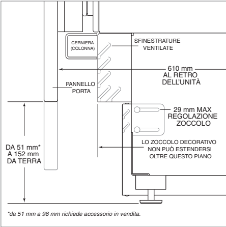
Area dello zoccolo (vista laterale).
