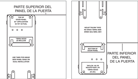
Plantilla del panel de la puerta: parte superior. Plantilla del panel de la puerta: parte inferior (modelo alto).
