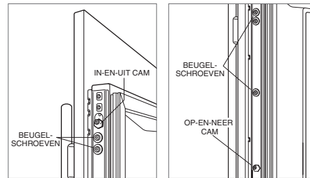
Aanpassing in-en-uit.
